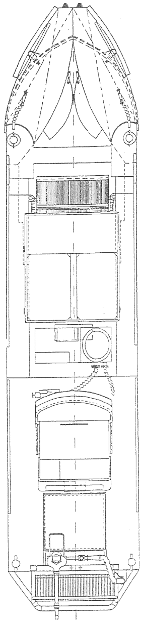
PLANTA CUBIERTA
