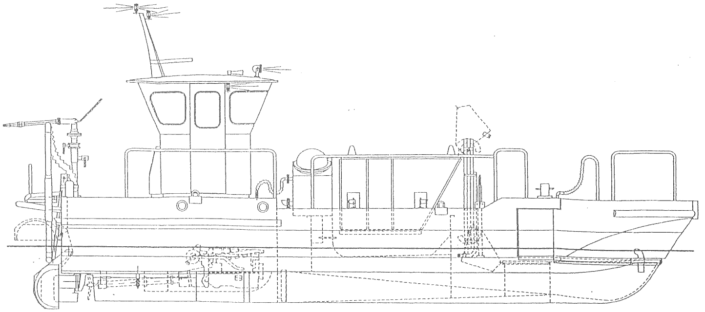
ALZADO LATERAL
